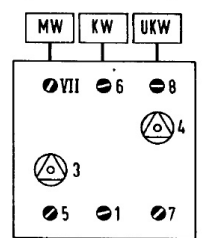
AM-Spulensatz von unten gesehen
