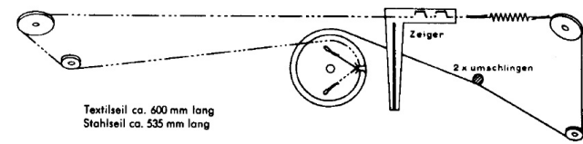
AM-Antrieb von der Skalen Seite gesehen
