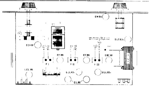
Chassis von oben gesehen
